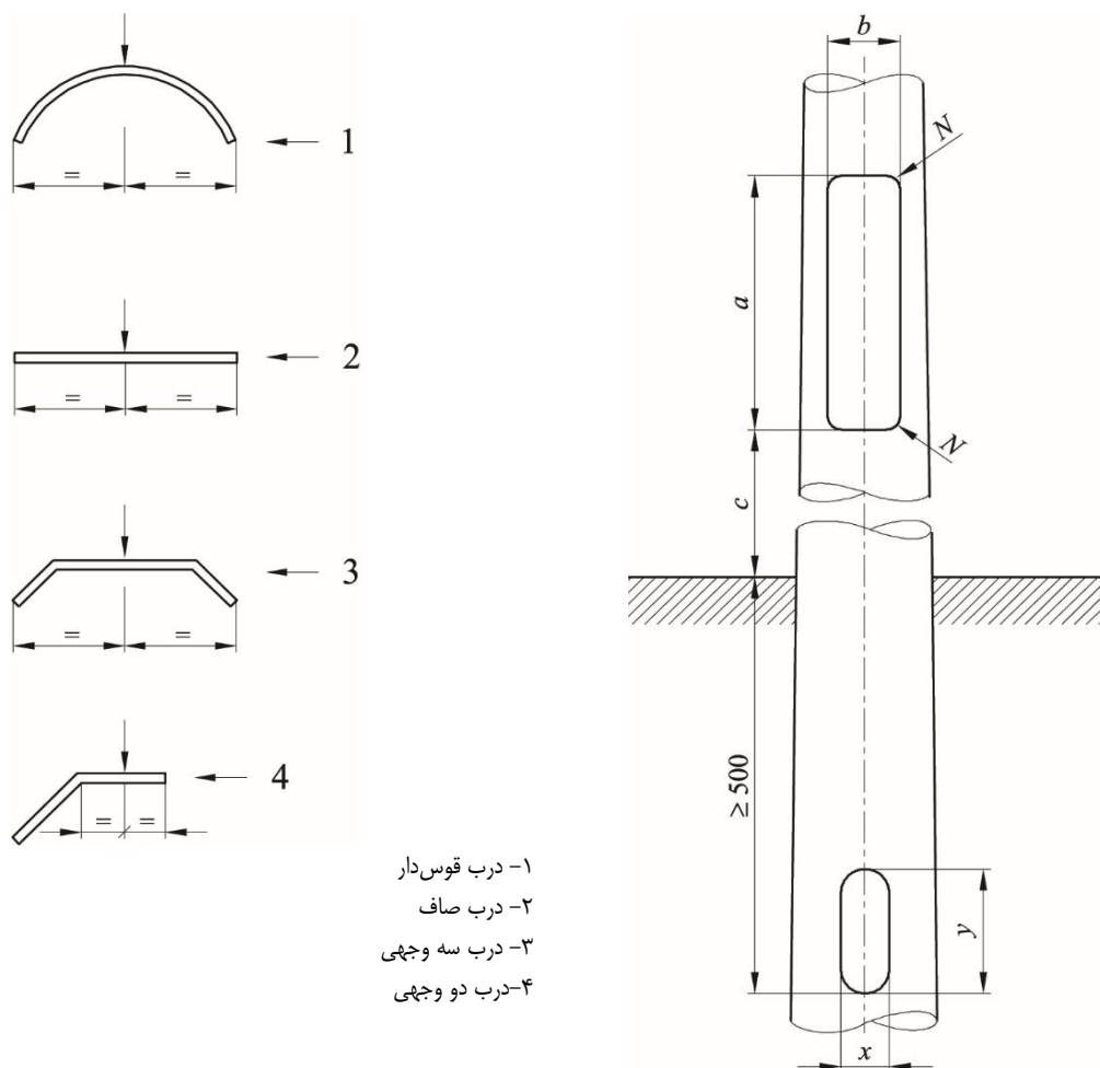
شکل ۸-۹: نمای مقابل برای آزمون ضربه دریچه
