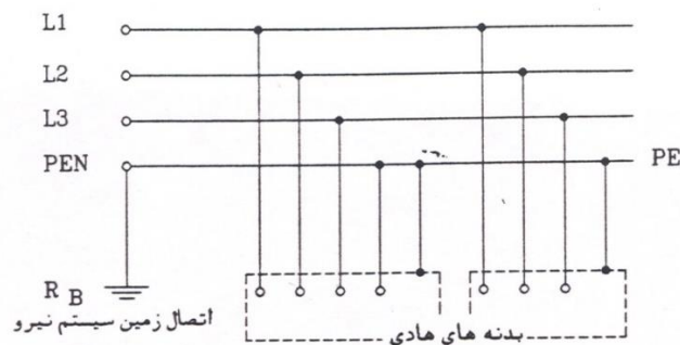
شکل ۱۰-۵: سیستم زمین نوع TN-C
