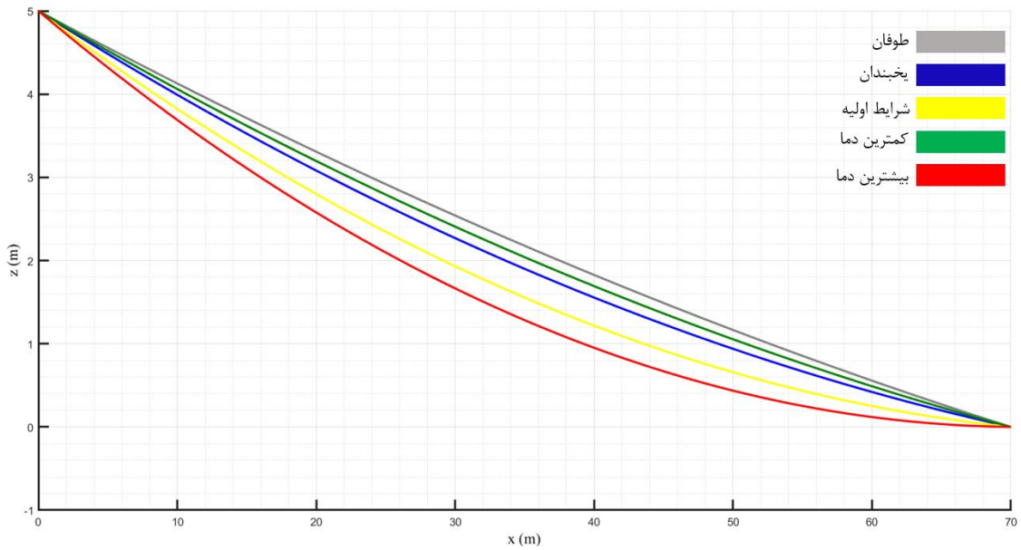
شکل ۲۰: منحنی سیم اسپن‌های ۴-۳ و ۵-۴ در صفحه z-x
