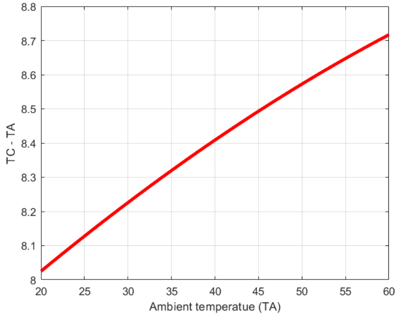
شکل ۱۶: اختلاف درجه حرارت هادی TC و درجه حرارت محیط TA برحسب تغییرات دمای محیط با هادی با جریان ۱۰۰ آمپر.
