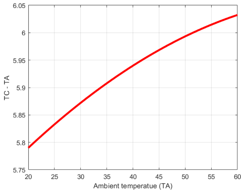
شکل ۱۷: اختلاف درجه حرارت هادی TC و درجه حرارت محیط TA برحسب تغییرات دمای محیط با هادی با جریان ۰ آمپر.
